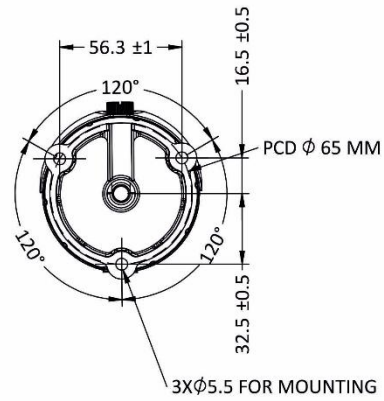
GSKT IPC BULLET REAR SILICON Ø56XØ4
